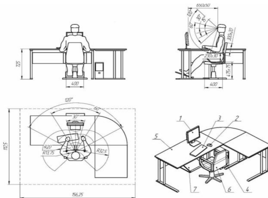
Рисунок 1. Графическое изображение рабочего места участника для всех основных нозологий (1. Монитор. 2. Мышь. 3. Клавиатура. 4. Подставка для ног. 5. Стол компьютерный. 6. Компьютерное кресло. 7. Подставка под клавиатуру).
