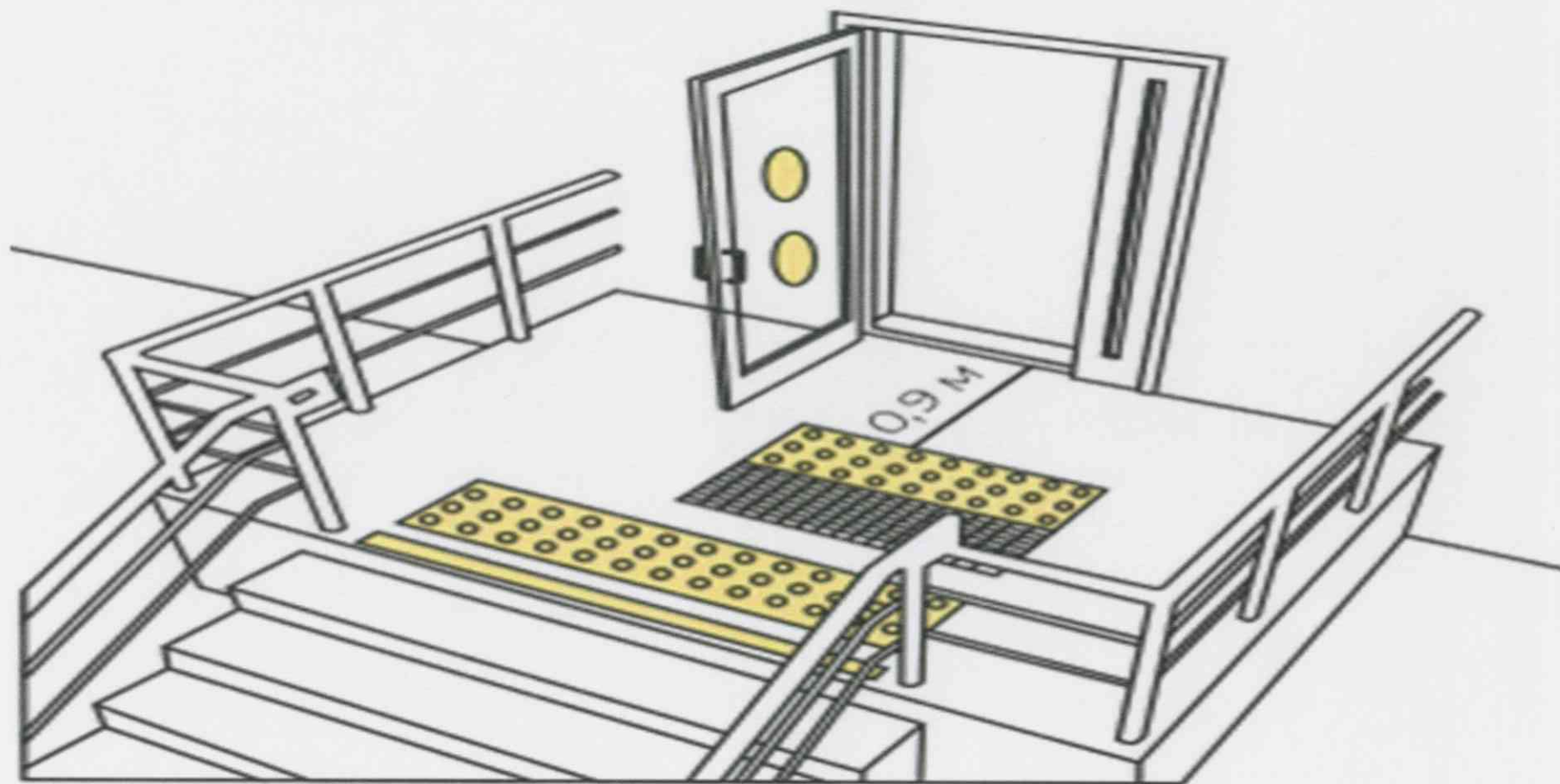
Тактильные указатели на входной площадке доступного входа.
