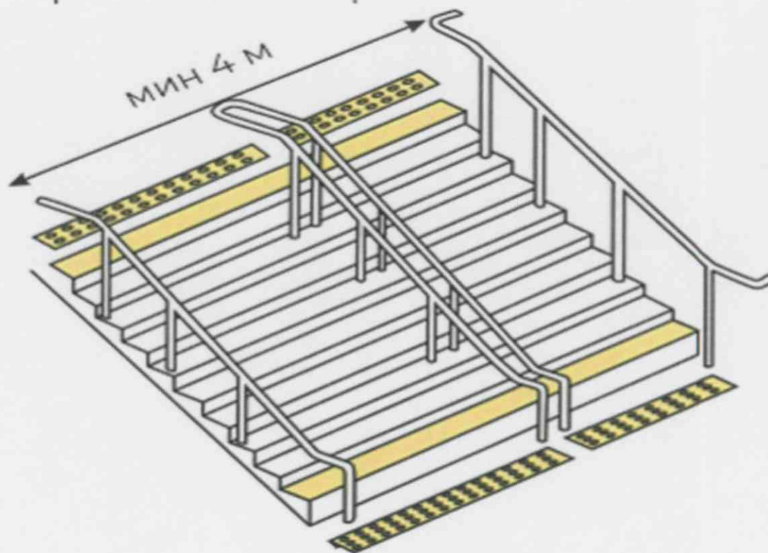
Устройство поручней на широкой наружной лестнице
