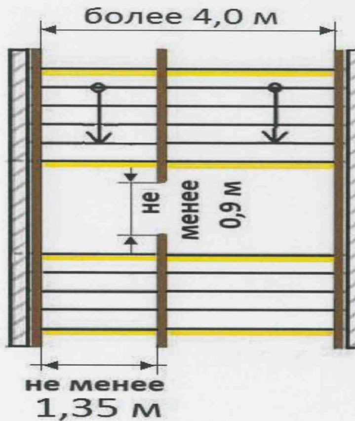
Устройство поручней на широкой наружной лестнице
