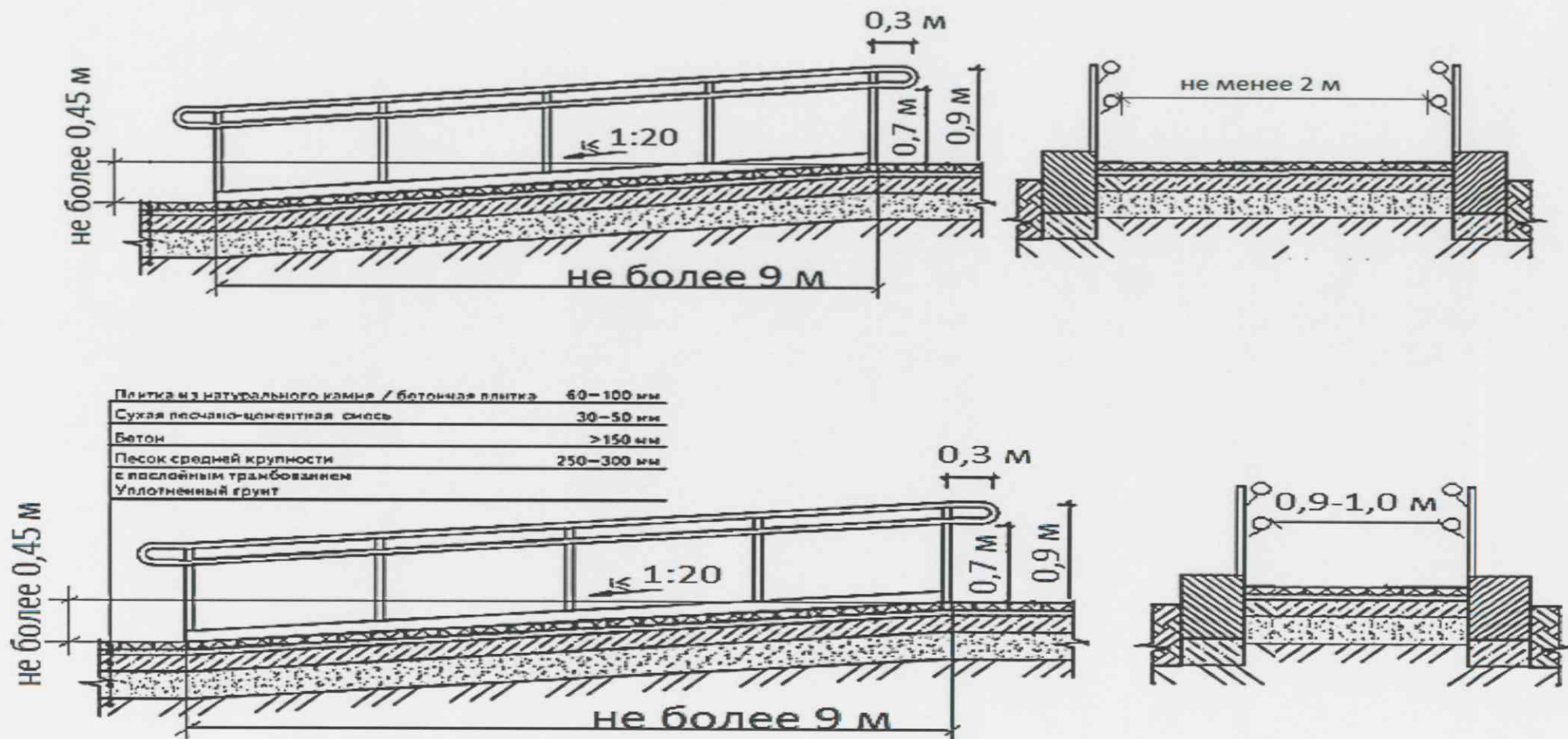
Стационарный пандус одностороннего движения
